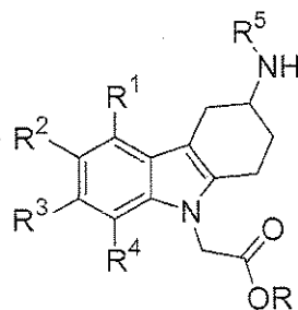
Structure 2a: R 5 ≠ H
