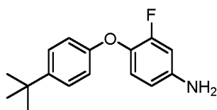
4-(4-(tert-butyl)phenoxy)-3-fluoroaniline,
