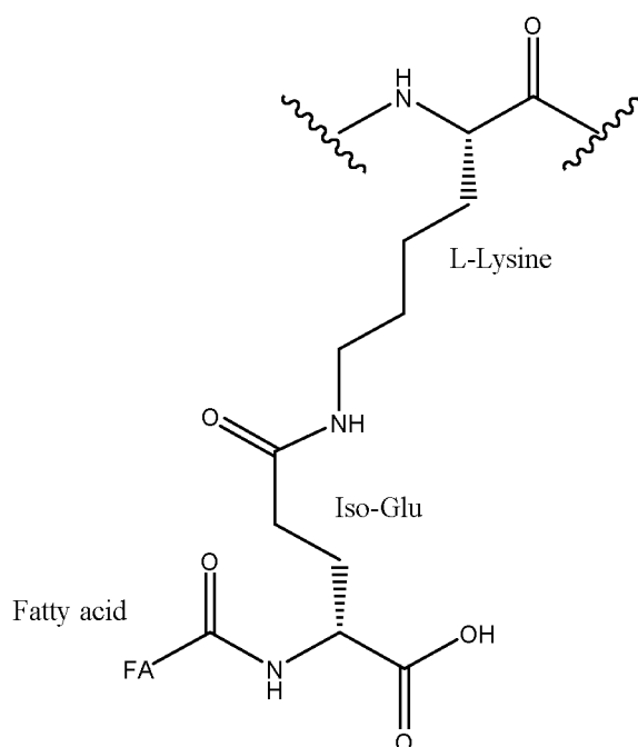
[K([Fatty acid]-isoGlu)]
