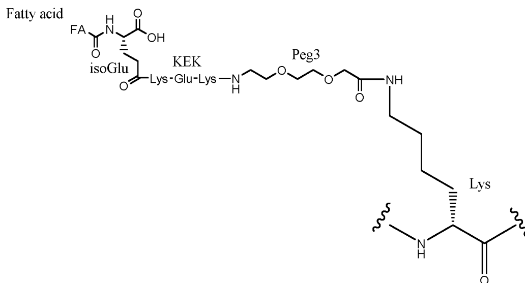
[K([Fatty acid]-isoGlu-KEK-Peg3)]
