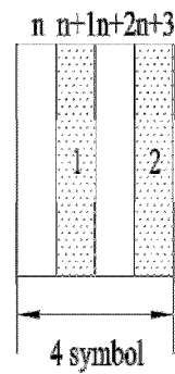
(b) n+1, n+3 symbol의 SRS 전송 할당 예
