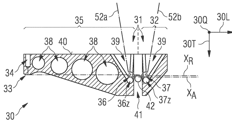
FIG 4 B-B
