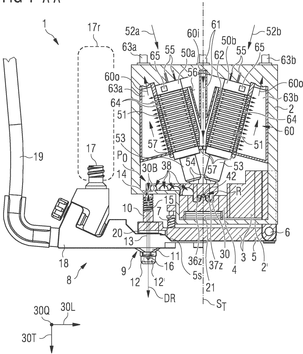
FIG 1 A-A
