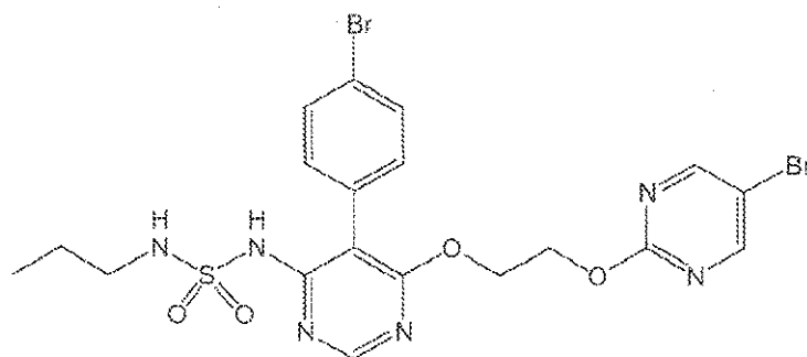
Macitentan
