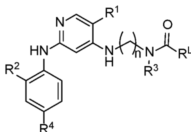
Formula IC
