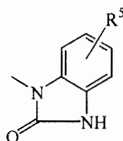
(b-11)
