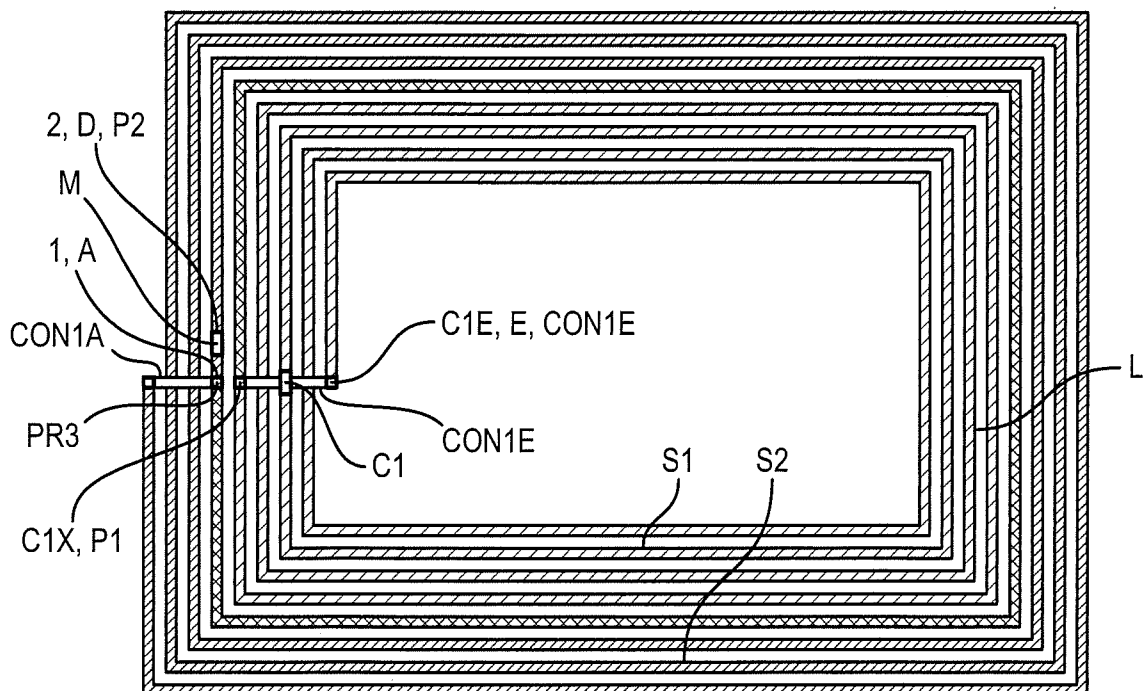
Antenna - 21AA
