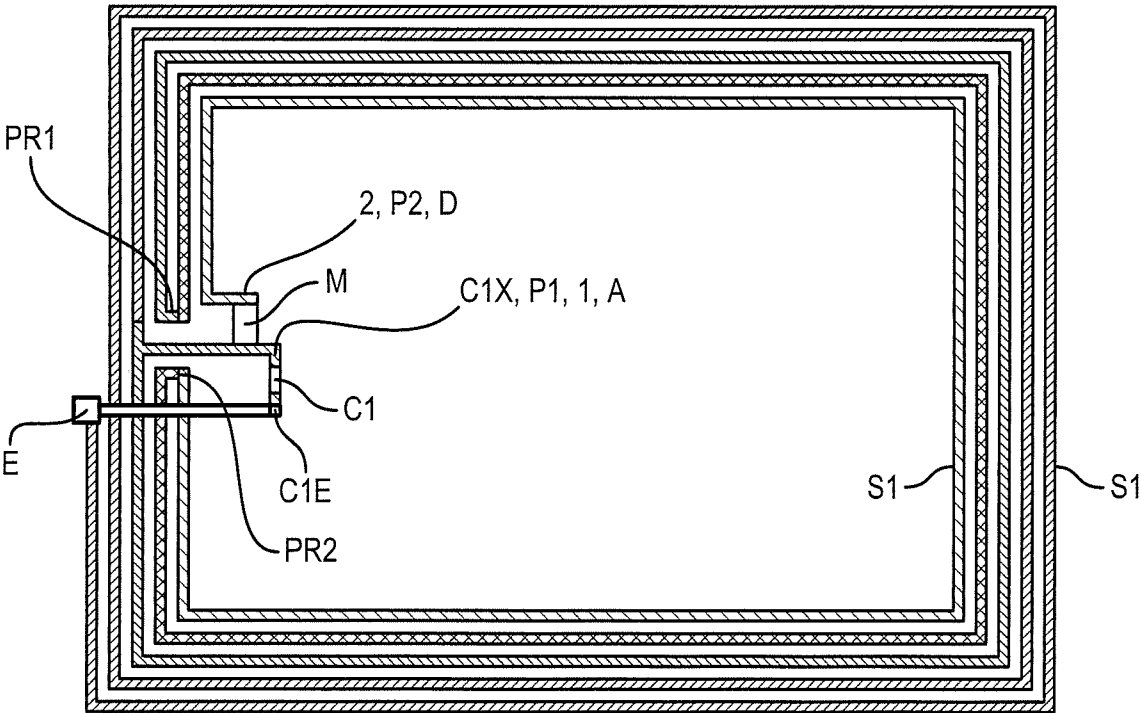
Antenna - 7
