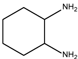
cyclohexane-1,2-diamine
