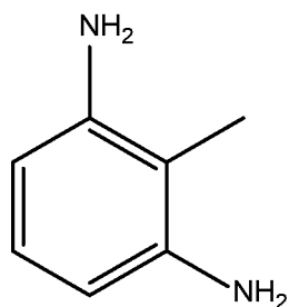
2,6-diaminotoluene
