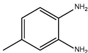
3,4-diaminotoluene
