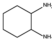
Cyclohexane-1,2-diamine
