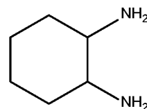
cyclohexane-1,2-diamine
