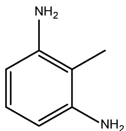
2,6-diaminotoluene
