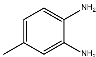
3,4-diaminotoluene
