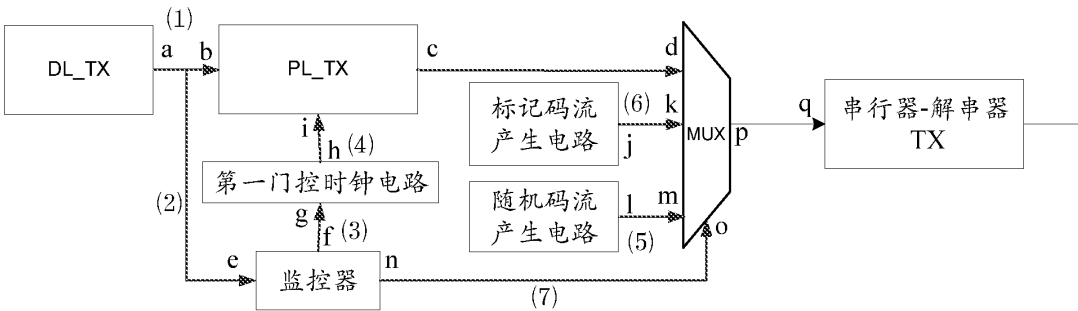
发送端的高速串行接口系统
