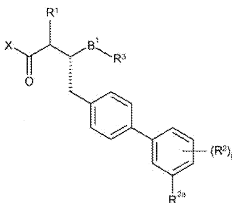
Formula IC
