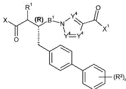
Formula VA
