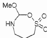
Compound D2
