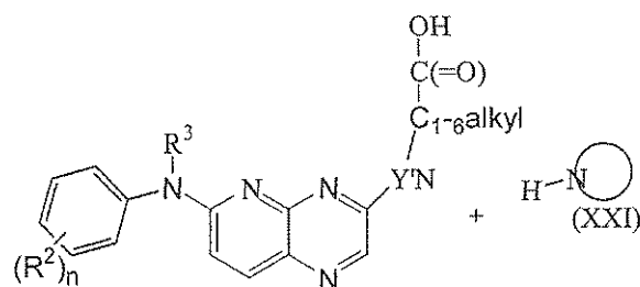
(XXIX)
