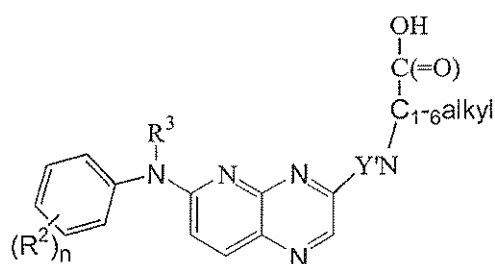
(XXIX)
