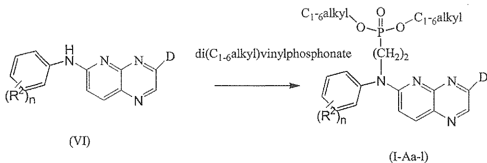
Scheme 1E
