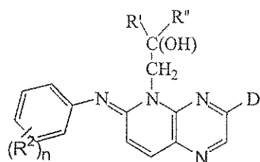
(I-Bb)
