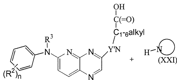
(XXIX)
