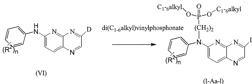
Scheme 1E
