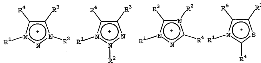
1,2,4-TRIAZOLIUM
