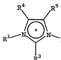
IMIDAZOLIUM
