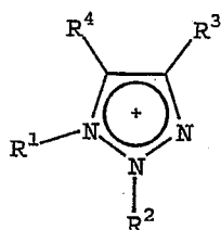
1,2,3-TRIAZOLIUM
