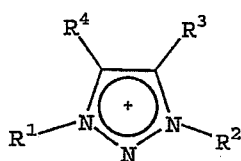
1,2,3-TRIAZOLIUM
