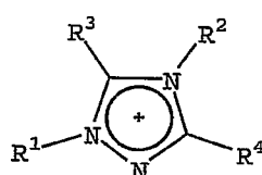
1,2,4-TRIAZOLIUM
