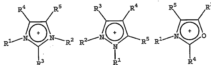
OXAZOLIUM
