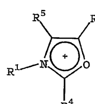
OXAZOLIUM
