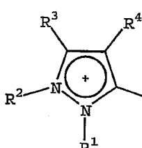
PYRAZOLIUM
