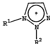
1,2,3-TRIAZOLIUM
