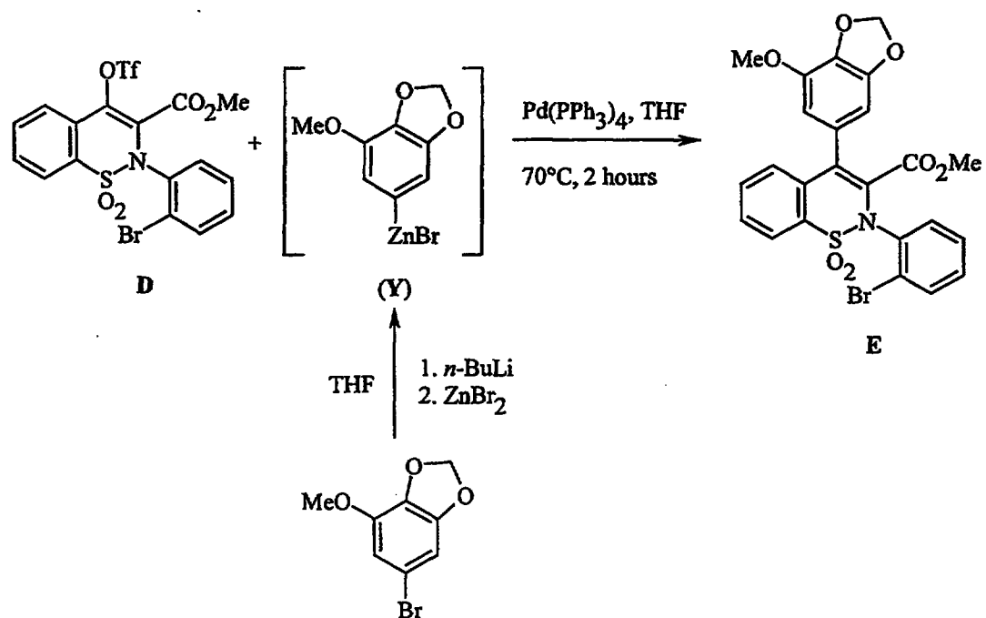
Scheme 1a
