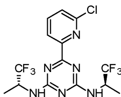
Vorasidenib
