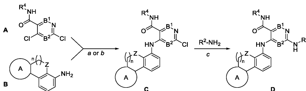
Scheme A:
