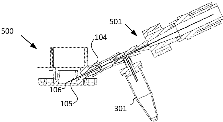
Fig. 7 A-A
