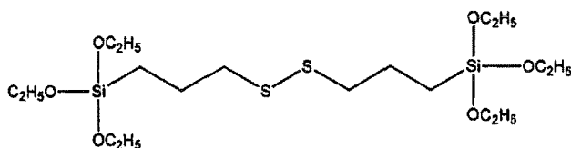
4,4,13,13-tetraethoxy-3,14-dioxa-8,9-dithia-4,13-disilahexadecane
