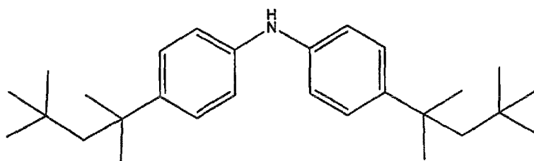
bis(4-(2,4,4-trimethylpentan-2-yl)phenyl)amine
