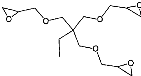
2,2'-(((2-ethyl-2-((oxiran-2-ylmethoxy)methyl)propane-1,3-diyl)bis(oxy))bis(methylene))bis(oxirane)
