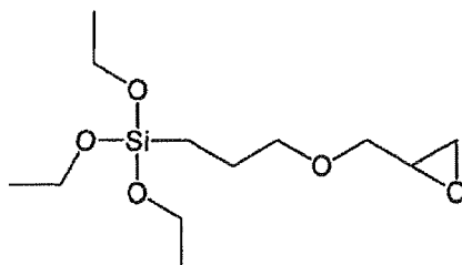
triethoxy(3-(oxiran-2-ylmethoxy)propyl)silane
