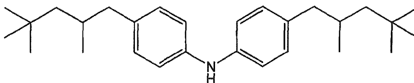
bis(4-(2,4,4-trimethylpentyl)phenyl)amine
