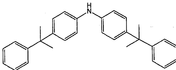
bis(4-(2-phenylpropan-2-yl)phenyl)amine
