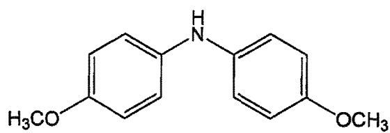
bis(4-methoxyphenyl)amine
