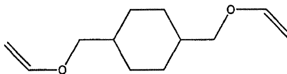
1,4-Bis[(ethenyloxy)methyl]-cyclohexane
