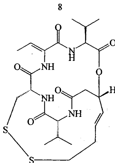
FR901228
