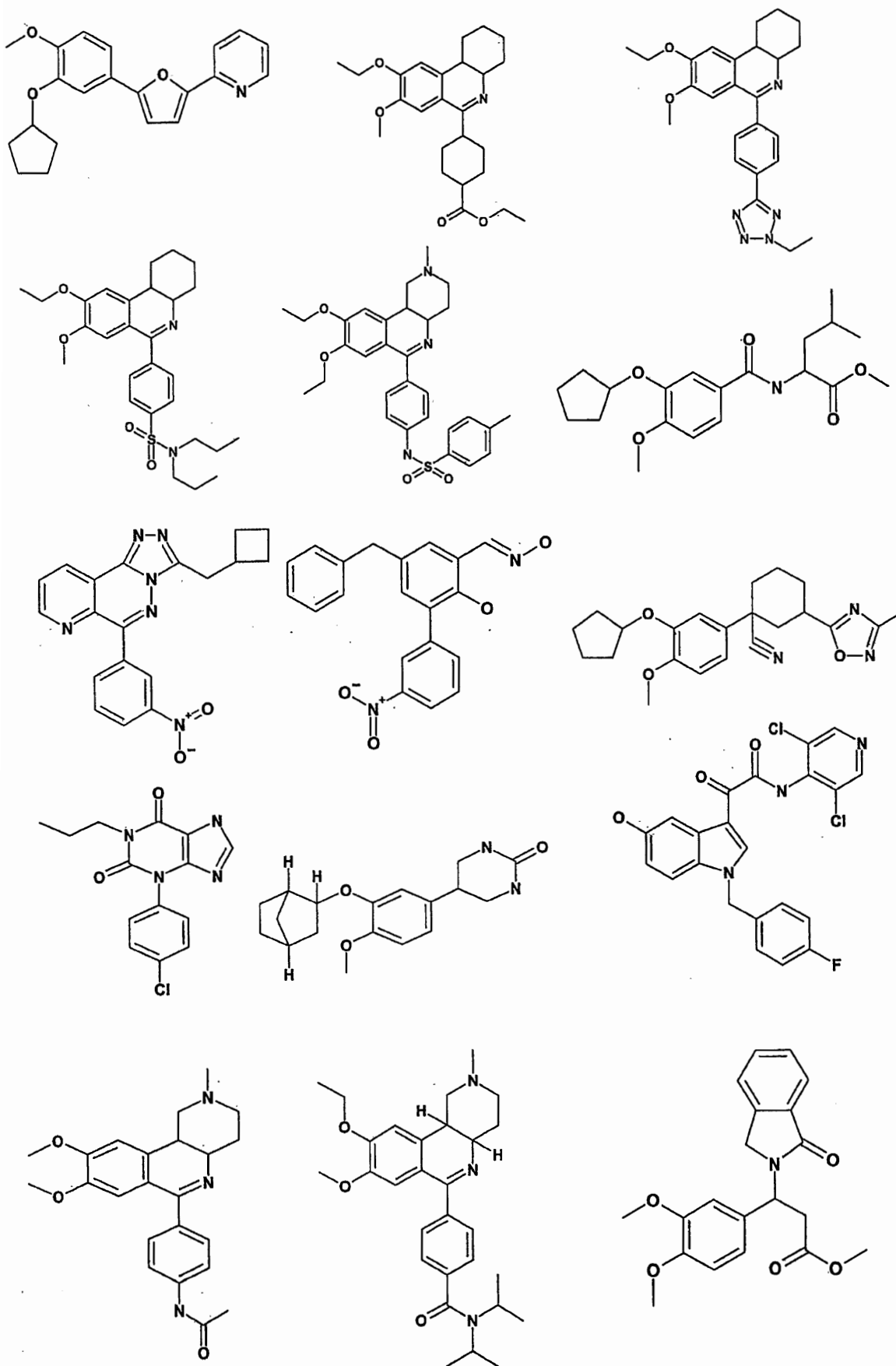
(Pumafentrin)
