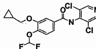
Roflumilast
