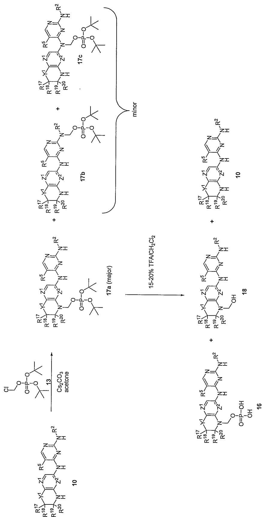
Scheme (IV)
