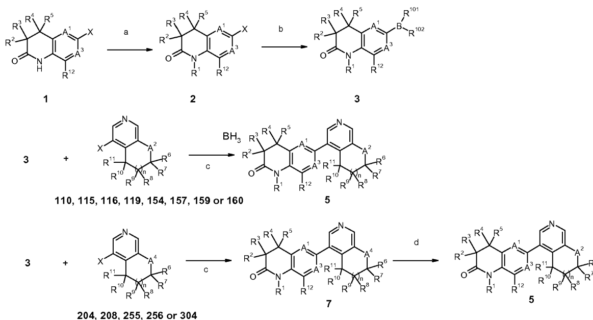
Scheme 1a
