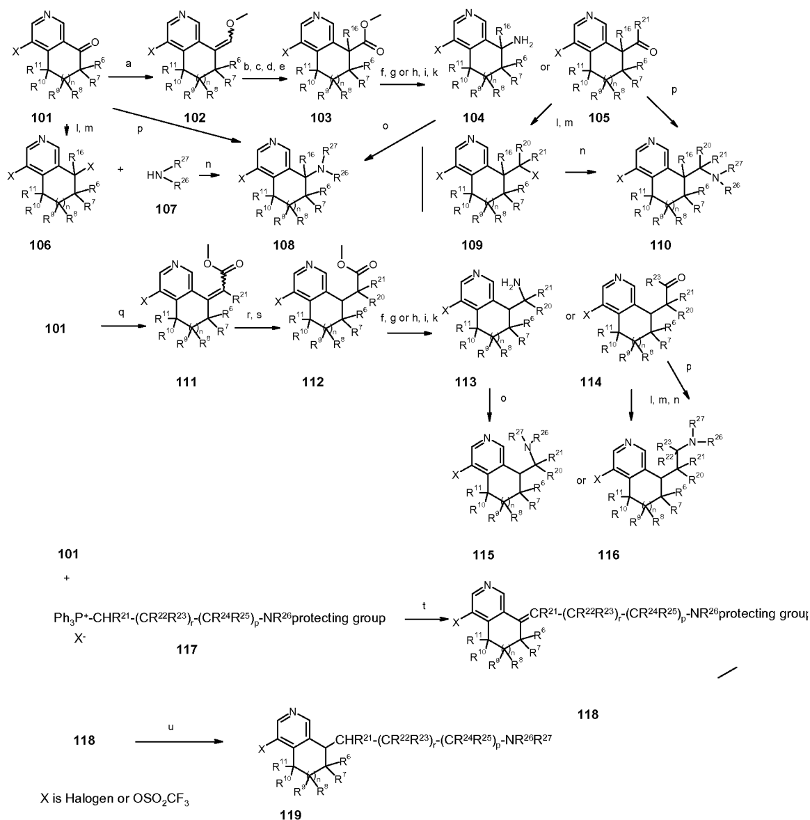
Scheme 2a
