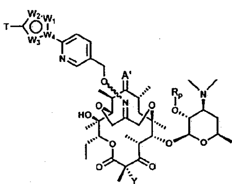
(XIV)
