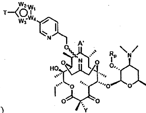
(XV)
