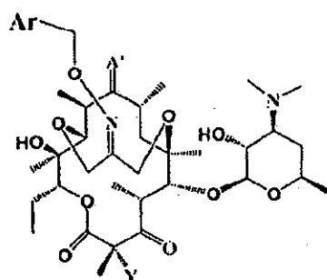
(XVI)
