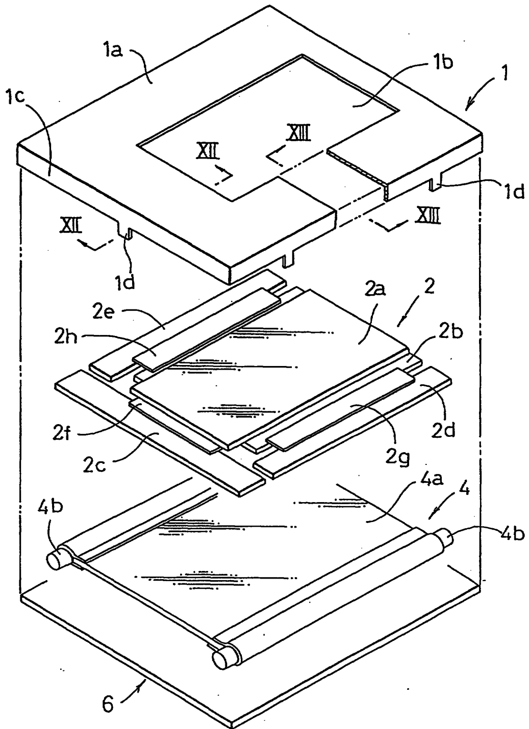
Fig.11(Prior Art)
