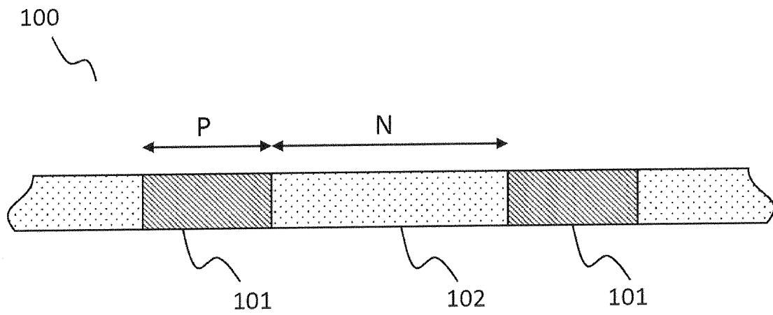
Prior art Fig. 1a
