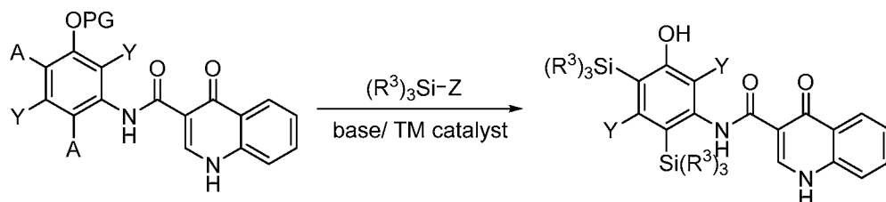
5 Scheme IV:
