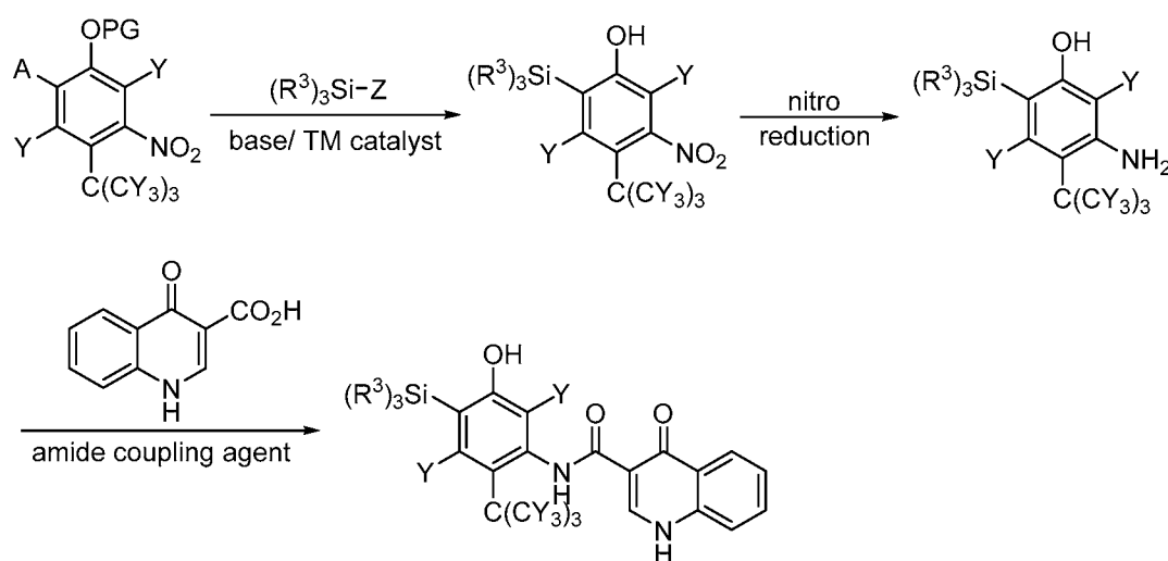
Scheme I:
