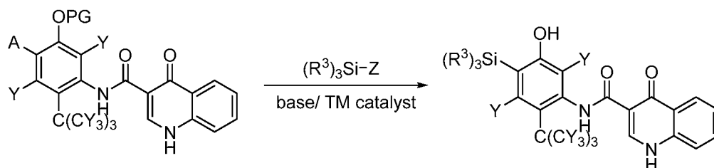
Scheme III:
