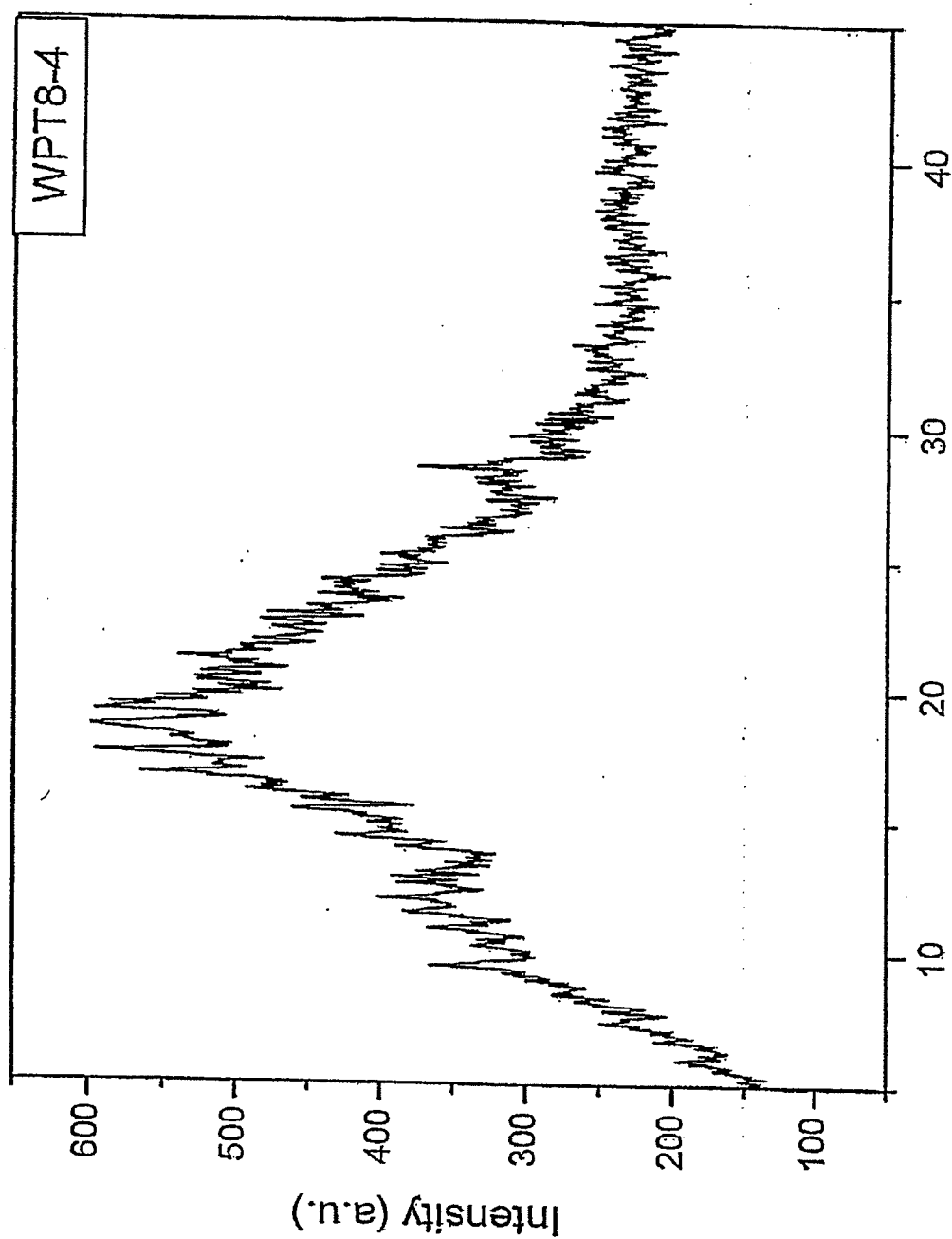
FIG. 8 2θ (degree)
