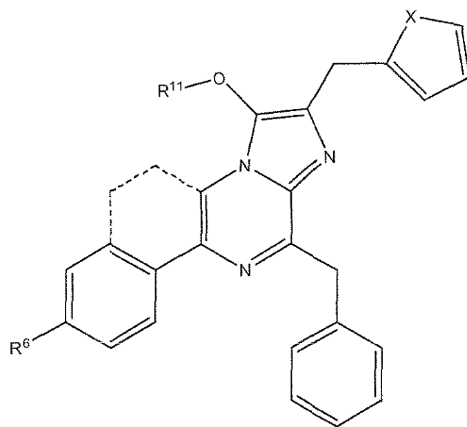
(IIb)
