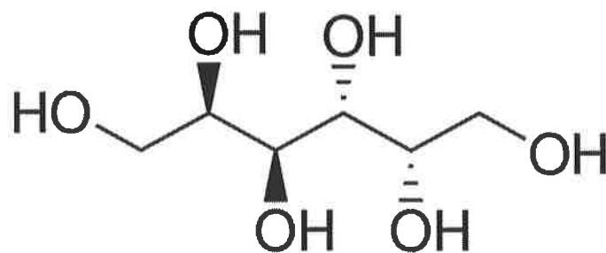
Dulcitol.
