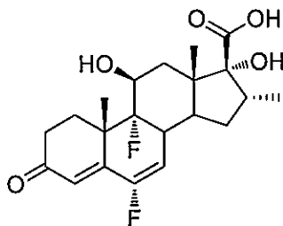
2-E
