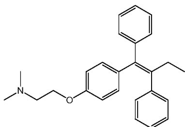
tamoxifen
