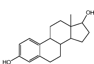
estradiol
