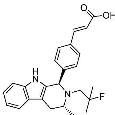
WO 2014/191726 Example 2
