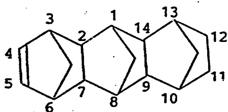
Hexacyclo[6,6,1,1 3.6 ,1 10.13 , 0 2.7 ,0 9.14 ]-4-heptadecene
