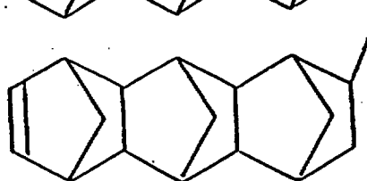
12-Isobutylhexacyclo[6,6,1,1 3.6 , 1 10.13 ,0 2.7 ,0 9.14 ]-4-heptadecene
