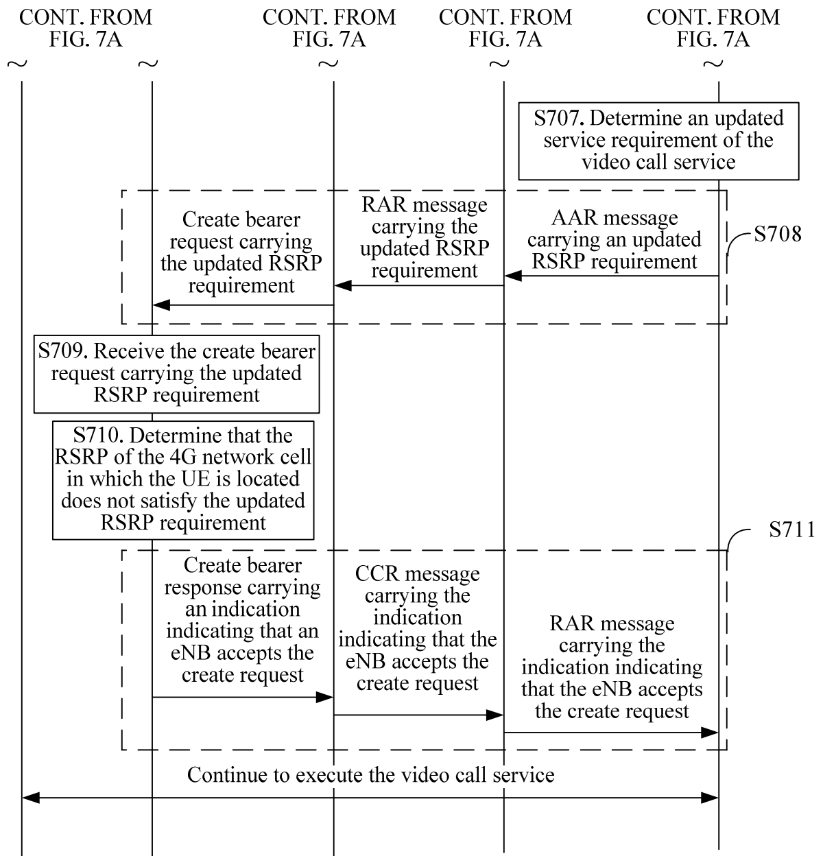
FIG. 7B
