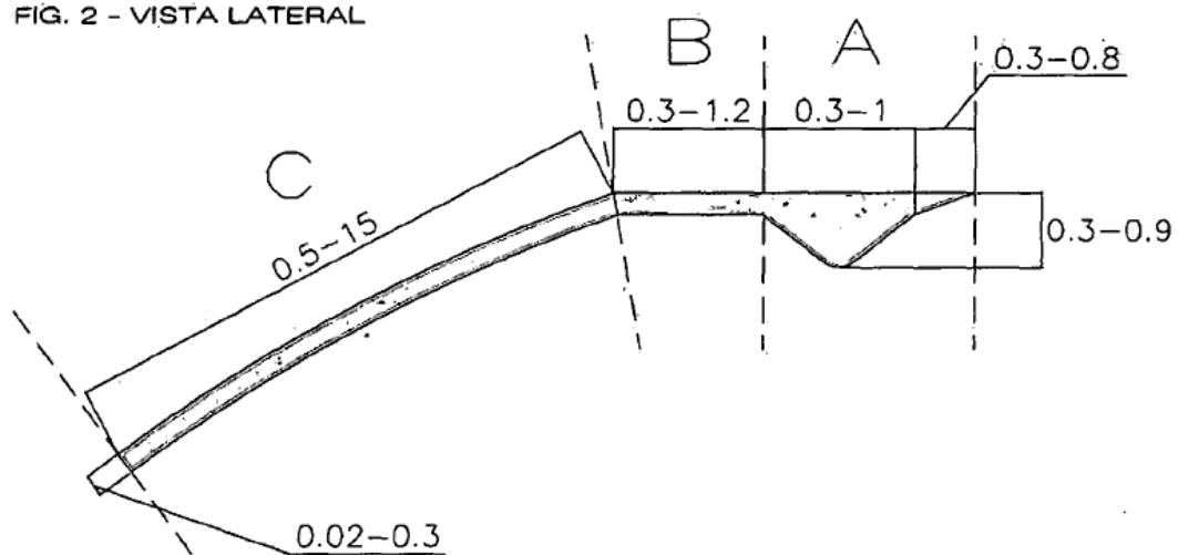
FIG. 2 - VISTA LATERAL
