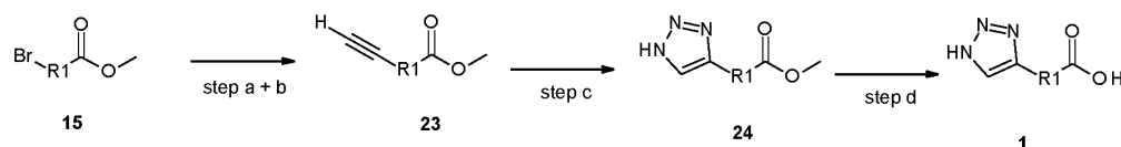
Scheme 9e
