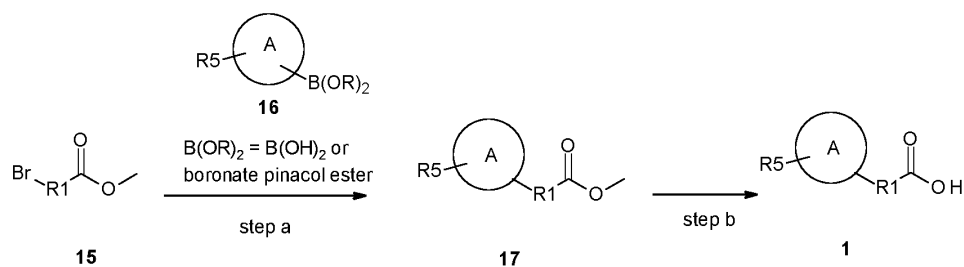
Scheme 9a
