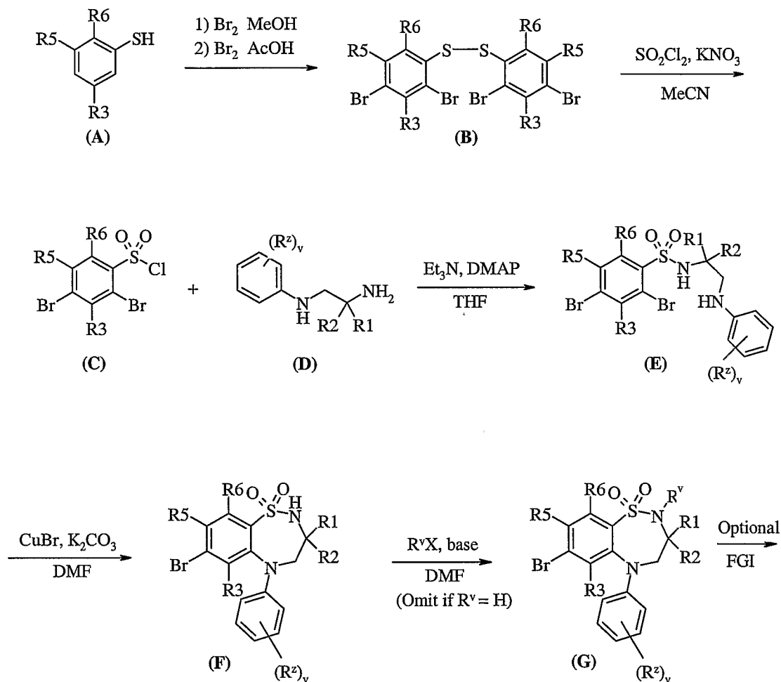
Scheme 1a
