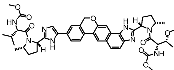
methyl [(2S)-1-{(2S,5S)-2-[5-(2-{(2S,5S)-1-[N-(methoxycarbonyl)-O-methyl-L-threonyl]-5-methylpyrrolidin-2-yl)-1,11-dihydroisochromeno[4',3':6,7]naphtho[1,2-d]imidazol-9-yl)-1H-imidazol-2-yl]-5-methylpyrrolidin-1-yl}-3-methyl-1-oxobutan-2-yl]carbamate
