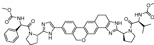
methyl [1-(2-{5-[2-(1-((methoxycarbonyl)amino)-3-methyl-1-oxobutan-2-yl)pyrrolidin-2-yl]-1,4,5,11-tetrahydroisochromeno[4',3':6,7]naphtho[1,2-d]imidazol-9-yl]-1H-imidazol-2-yl)pyrrolidin-1-yl)-phenyl-1-oxoacet-2-yl]carbamate
