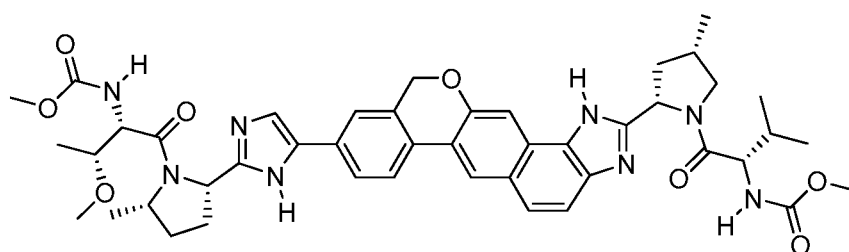
methyl [(2S)-1-((2S,4S)-2-[9-(2-((2S,5S)-1-[N-(methoxycarbonyl)-O-methyl-L-threonyl]-5-methylpyrrolidin-2-yl)-1H-imidazol-5-yl)-1,11-dihydroisochromeno[4',3':6,7]naphtho[1,2-d]imidazol-2-yl]-4-methylpyrrolidin-1-yl]-3-methyl-1-oxobutan-2-yl]carbamate
