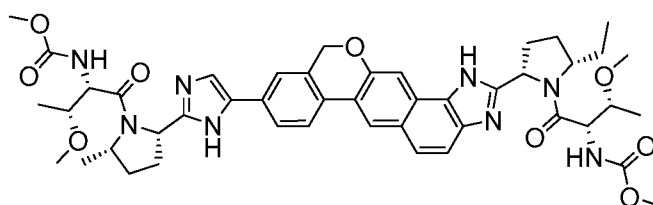
methyl[(2S,3R)-1-{(2S,5S)-2-[5-(2-{(2S,5S)-5-ethyl-1-[N-(methoxycarbonyl)-O-methyl-L-threonyl]pyrrolidin-2-yl)-1,11-dihydroisochromeno[4',3':6,7]naphtho[1,2-d]imidazol-9-yl)-1H-imidazol-2-yl]-5-methylpyrrolidin-1-yl]-3-methoxy-1-oxobutan-2-yl]carbamate
