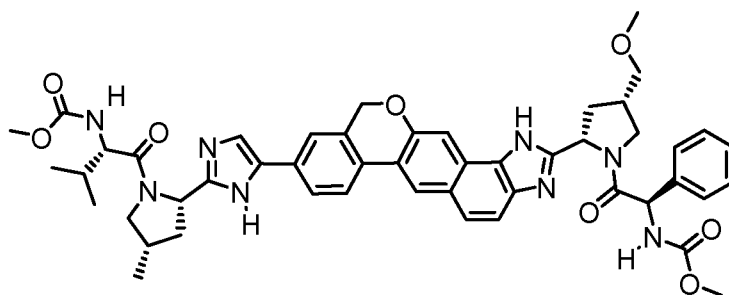
methyl ((2S)-1-((2S,4S)-2-(5-bromo-1H-imidazol-2-yl)-4-methylpyrrolidin-1-yl)-3-methyl-1-oxobutan-2-yl)carbamate
