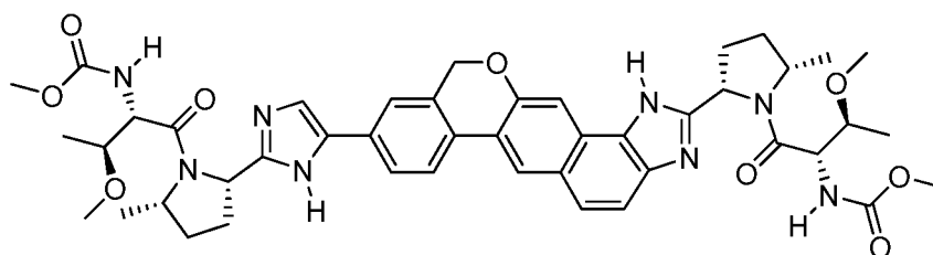
methyl [(2S,3S)-3-methoxy-1-{(2S,5S)-2-[9-(2-{(2S,5S)-1-[N-(methoxycarbonyl)-O-methyl-L-allothreonyl]-5-methylpyrrolidin-2-yl]-1H-imidazol-5-yl)-1,11-dihydroisochromeno[4',3':6,7]naphtho[1,2-d]imidazol-2-yl]-5-methylpyrrolidin-1-yl}-1-oxobutan-2-yl]carbamate
