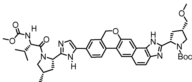
tert-butyl (2S,4S)-2-[9-(2-((2S,4S)-1-[N-(methoxycarbonyl)-L-valyl]-4-methylpyrrolidin-2-yl)-1H-imidazol-5-yl)-3,11-dihydroisochromeno[4',3':6,7]naphtho[1,2-d]imidazol-2-yl]-4-(methoxymethyl)pyrrolidine-1-carboxylate
