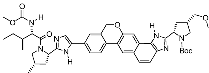
tert-butyl (2S,4S)-2-[9-(2-((2S,4S)-1-[N-(methoxycarbonyl)-L-alloisoleucyl]-4-methylpyrrolidin-2-yl)-1H-imidazol-5-yl)-1,11-dihydroisochromeno[4',3':6,7]naphtho[1,2-d]imidazol-2-yl]-4-(methoxymethyl)pyrrolidine-1-carboxylate
