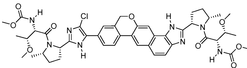
methyl [(2S,3R)-1-((2S,5S)-2-[9-(4-chloro-2-((2S,5S)-1-[N-(methoxycarbonyl)-O-methyl-L-threonyl]-5-methylpyrrolidin-2-yl)-1H-imidazol-5-yl)-1,11-dihydroisochromeno[4',3':6,7]naphtho[1,2-d]imidazol-2-yl]-5-methylpyrrolidin-1-yl)-3-methoxy-1-oxobutan-2-yl]carbamate
