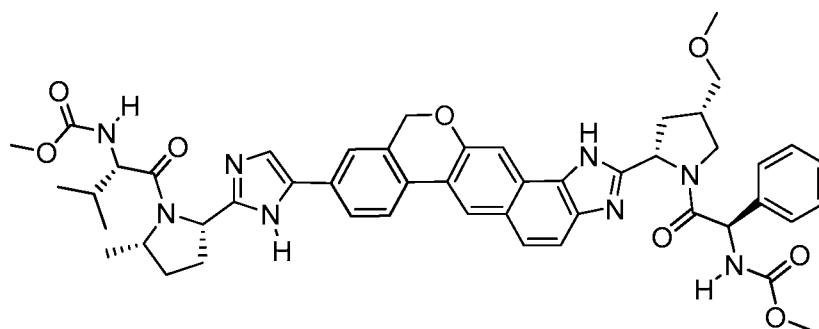
Methyl {(2S)-1-[(2S,5S)-2-(5-{2-[(2S,4S)-1-[(2R)-2-[(methoxycarbonyl)amino]-2-phenylacetyl]-4-(methoxymethyl)pyrrolidin-2-yl]-1,11 dihydroisochromeno [4',3':6,7]naphtho[1,2-d]imidazol-9-yl}-1H-imidazol-2-yl)-5-methylpyrrolidin-1-yl]-3-methyl-1-oxobutan-2-yl} carbamate
