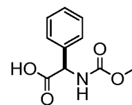
(R)-2-(methoxycarbonylamino)-2-phenylacetic acid
