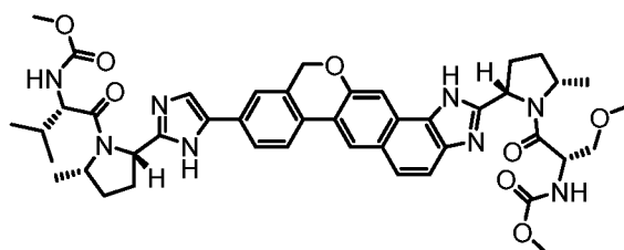
methyl [(2S)-1-{(2S,5S)-2-[5-(2-{(2S,5S)-1-[N-(methoxycarbonyl)-O-methyl-L-seryl]-5-methylpyrrolidin-2-yl)-1,11-dihydroisochromeno[4',3':6,7]naphtho[1,2-d]imidazol-9-yl)-1H-imidazol-2-yl]-5-methylpyrrolidin-1-yl}-3-methyl-1-oxobutan-2-yl]carbamate
