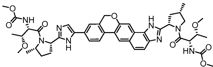
methyl [(2S,3R)-3-methoxy-1-[(2S,5S)-2-[9-(2-{(2S,5S)-1-[N-(methoxycarbonyl)-O-methyl-L-threonyl]-5-methylpyrrolidin-2-yl]-1H-imidazol-5-yl)-1,11-dihydroisochromeno[4',3':6,7]naphtho[1,2-d]imidazol-2-yl]-4-methylpyrrolidin-1-yl]-1-oxobutan-2-yl]carbamate
