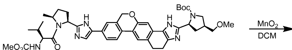
tert-butyl (2S,4S)-2-[9-(2-((2S,5S)-1-[N-(methoxycarbonyl)-L-valyl]-5-methylpyrrolidin-2-yl)-1H-imidazol-5-yl)-1,4,5,11-tetrahydroisochromeno[4',3':6,7]naphtho[1,2-d]imidazol-2-yl)-4-(methoxymethyl)pyrrolidine-1-carboxylate
