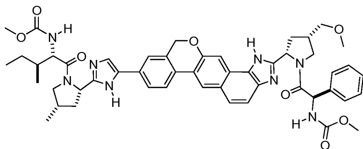
methyl ((1R)-2-[(2S,4S)-2-(9-{2-[(2S,4S)-1-((2S,3R)-2-[(methoxycarbonyl)amino]-3-methylpentanoyl)-4-methylpyrrolidin-2-yl]-1H-imidazol-5-yl)-1,11-dihydroisochromeno[4',3':6,7]naphtho[1,2-d]imidazol-2-yl)-4-(methoxymethyl)pyrrolidin-1-yl]-2-oxo-1-phenylethyl)carbamate
