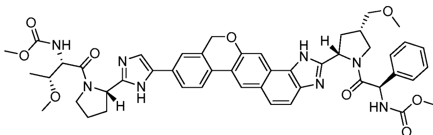
methyl {(1R)-2-[(2S,4S)-2-[9-(2-{(2S)-1-[(2S,3R)-3-methoxy-2-[(methoxycarbonyl)amino]butanoyl]pyrrolidin-2-yl]-1H-imidazol-5-yl)-1,11-dihydroisochromeno[4',3':6,7]naphtho[1,2-d]imidazol-2-yl]-4-(methoxymethyl)pyrrolidin-1-yl]-2-oxo-1-phenylethyl}carbamate
