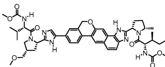
methyl {(2S,3S)-1-[(2S,5S)-2-(9-{2-[(2S,4S)-1-{(2S)-2-[(methoxycarbonyl)amino]-3-methylbutanoyl}-4-(methoxymethyl)pyrrolidin-2-yl]-1H-imidazol-5-yl}-1,11-dihydroisochromeno[4',3':6,7]naphtho[1,2-d]imidazol-2-yl)-5-methylpyrrolidin-1-yl]-3-methyl-1-oxopentan-2-yl}carbamate
