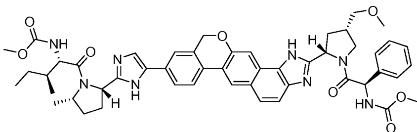
methyl {(1R)-2-[(2S,4S)-2-[9-(2-[(2S,5S)-1-[(2S,3S)-2-[(methoxycarbonyl)amino]-3-methylpentanoyl]-5-methylpyrrolidin-2-yl]-1H-imidazol-5-yl)-1,11-dihydroisochromeno[4',3':6,7]naphtho[1,2-d]imidazol-2-yl)-4-(methoxymethyl)pyrrolidin-1-yl]-2-oxo-1-phenylethyl}carbamate
