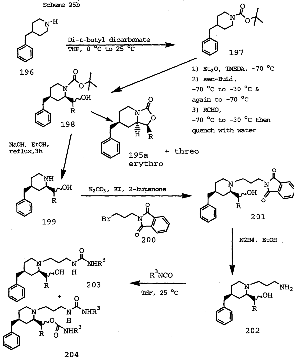
Scheme 25b
