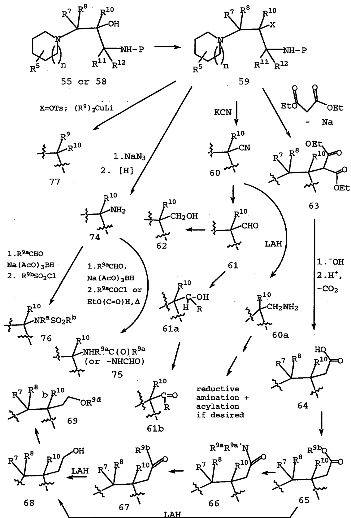
SCHEME 9 (con't)
