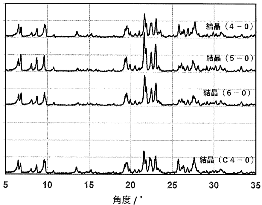
アルミノシリケートのXRDチャート
