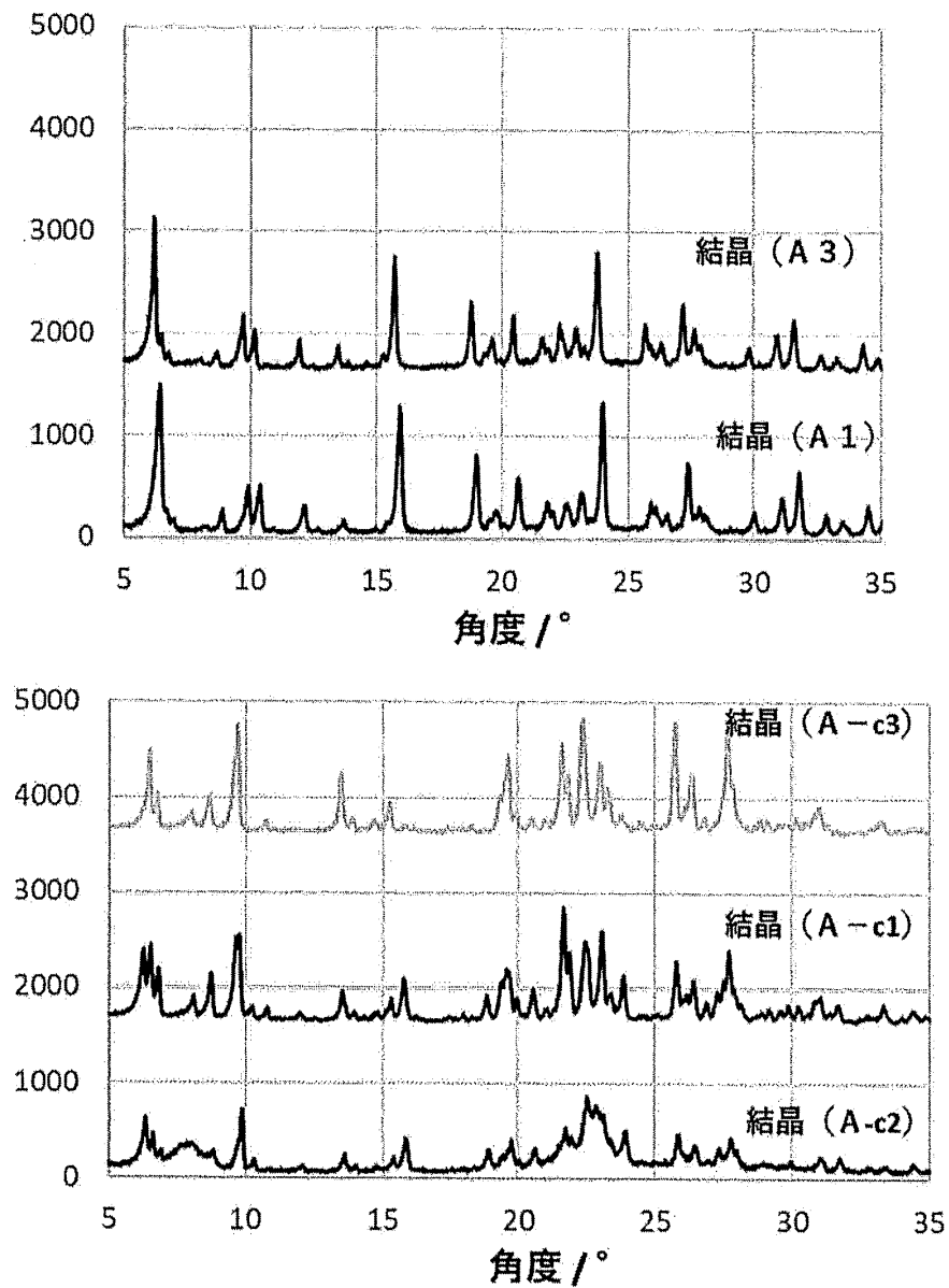
実施例、比較例の結晶 (A) のXRDチャート
