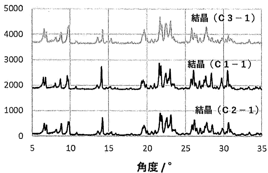
実施例、比較例のアルミノシリケートのXRDチャート
