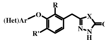
5: X = NH, O, S
