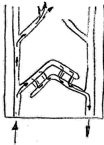
aufsteigende Spülrichtung
