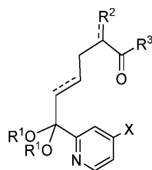
(IIa)
