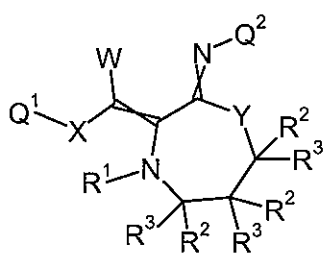
Formula 7.N.1
