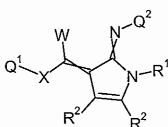
Formula 5.L.2
