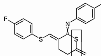
WO2011958963 Example 2-6
