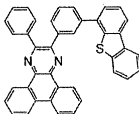
3Ph-2mDBTPDBq-II
