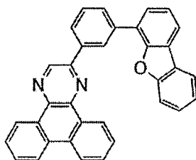
2mDBFPDBq-II
