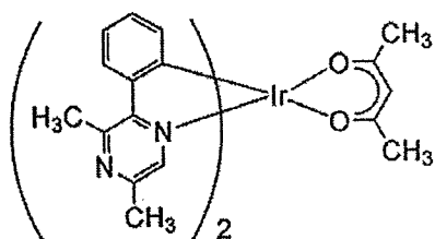
\text{Ir}(\text{mppr-Me})_2\text{acac}
