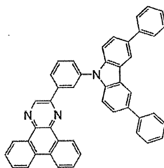
2mCzPDBq-III
