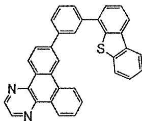
7mDBTPDBq-II
