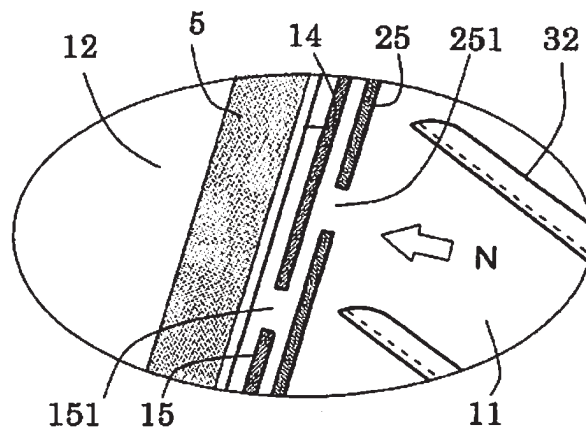
図1のL部拡大
