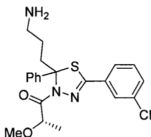
(2S)-1-(2-(3-Aminopropyl)-5-(3-chlorophenyl)-2-phenyl-1,3,4-thiadiazol-3(2H)-yl)-2-methoxypropan-1-one
