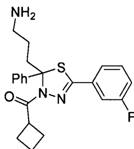
(2-(3-Aminopropyl)-5-(3-fluorophenyl)-2-phenyl-1,3,4-thiadiazol-3(2H)-yl)(cyclobutyl)methanone
