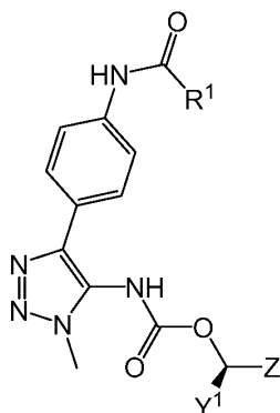
(IIj)
