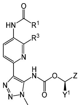
(IIe)
