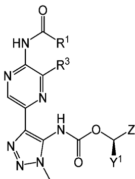
(IIh)
