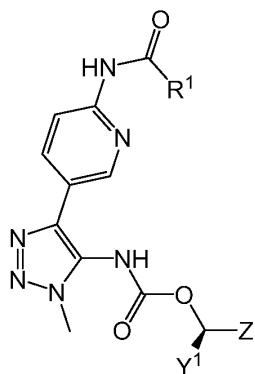
(III)
