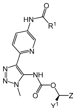
(II o )
