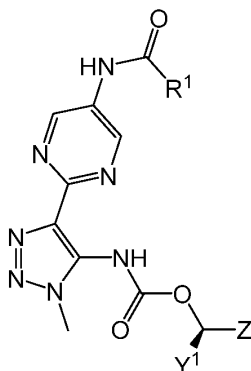
(IIk)
