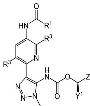
(IIg)
