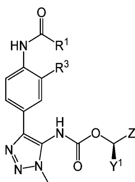
(IIa)
