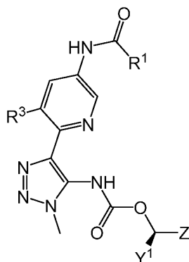
(II n )
