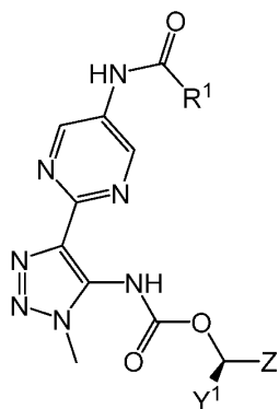
(IIk)
