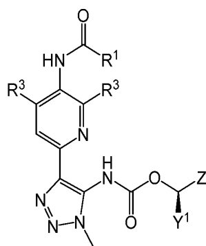
(IIf)
