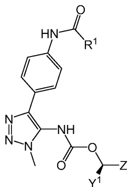
(IIj)
